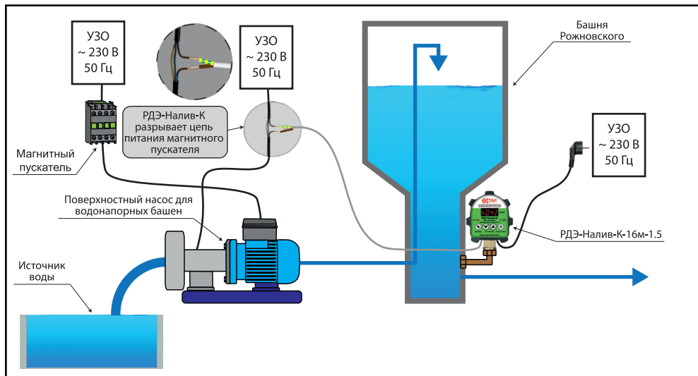
Пример 3. Пример подключения РДЭ-Налив-К-16м-1.5 для управления поверхностным насосом мощностью Р1 менее 1.5 кВт башни Рожновского.
