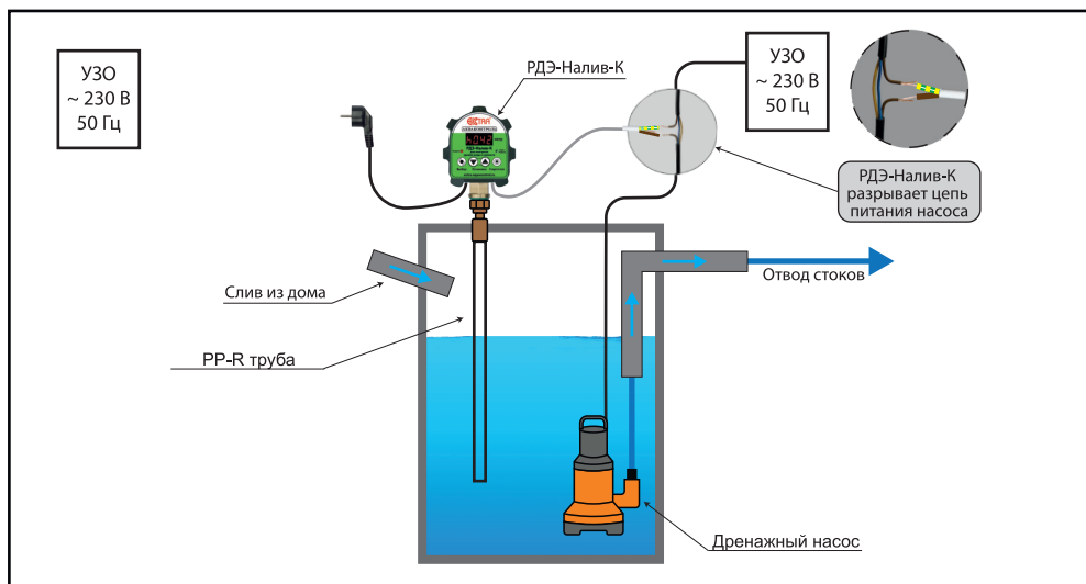
Пример 4. Подключение РДЭ-Налив-К в режиме СР-2 для управления дренажным насосом.
