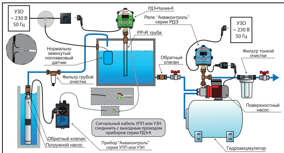
Пример 6. Обеспечение плавного пуска и защиты от сухого хода насоса установленного в малодебитной скважине при организации водоснабжения с использованием накопительной емкости.
