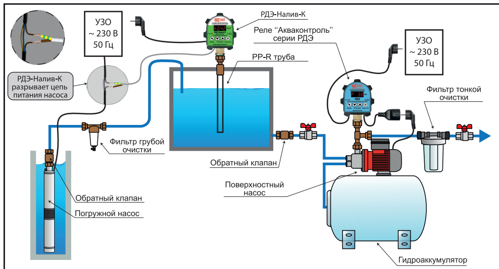
Пример 5. Подключение РДЭ-Налив-К в режиме СР-2 с наполняющим погружным и раздающим поверхностным насосом.
